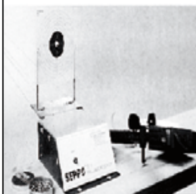
SEPPÖ H 96 TAULUNSIIRTOLAITE NYKYIAIKAINEN JA NOPEA TAULUN LIIKUTUKSEEN.
